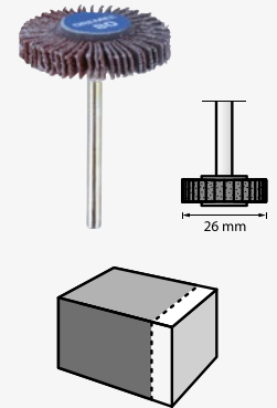
Schleiffächer 9,5 mm (502)
