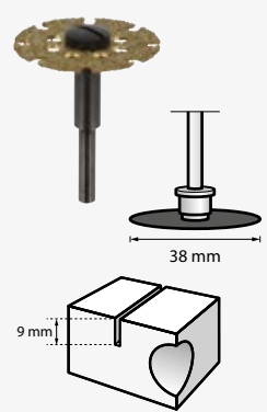
Disco de corte/ conformado 25,4 mm (542)
