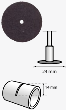
Disco de corte de 24 mm (409)
