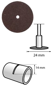
Disco de corte para trabajos duros de 24 mm (420)
