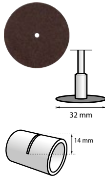
Disco de corte de 32 mm (540)
