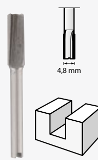
Fresa (HSS) 4,8 mm (652)
