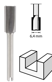
Fresa (HSS) 6,4 mm (654)
