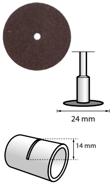
Disco da taglio Heavy Duty da 24 mm (420)
