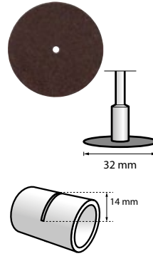
Snijschijf 32 mm (540)
