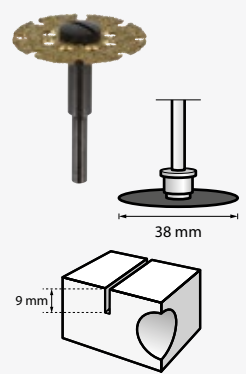
Frees/schaafschijf 25,4 mm (542)
