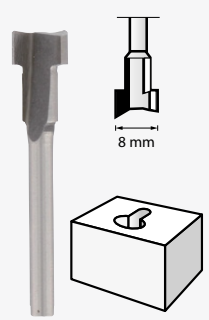
Frez do zarysów płaskich (HSS) 8,0 mm (655)
