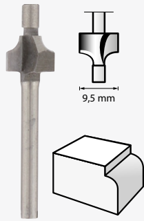
Frez do zarysów płaskich (HSS) 9,5 mm (612)
