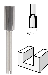
Frez do zarysów płaskich (HSS) 6,4 mm (654)
