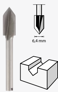
Резец для фасонно-фрезерного станка (HSS) 6,4 мм (640)
