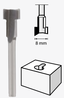
Резец для фасонно-фрезерного станка (HSS) 8,0 мм (655)
