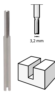
Резец для фасонно-фрезерного станка (HSS) 3,2 мм (650)
